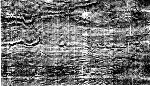
Şekil 7. Bir yanar sonar mozaiği, A: kaya mostraları ve yer yer riflerin olduğu siltli bölge, B: rif toplulukları, C: volkanik kıvrımlar, D: killle kaplı düz deniz tabanı, ortalama derinlik: 450 m.
